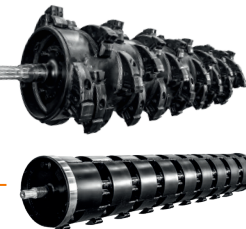
固定齿刀鼓 (UML) 或 摆锤式刀鼓 (FML)
